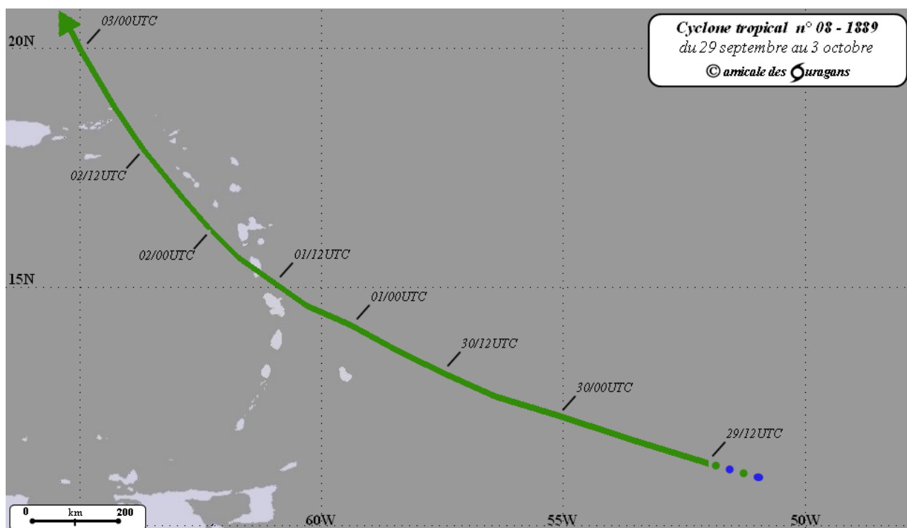
Trajectoire officielle du centre du cyclone n° 8 du 29 septembre au 3 octobre 1889
