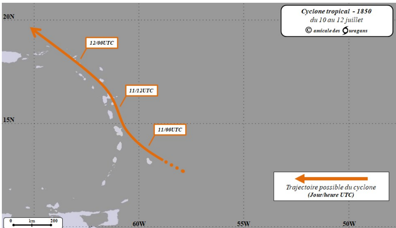
Trajectoire possible du centre du cyclone du 10 au 12 juillet 1850
