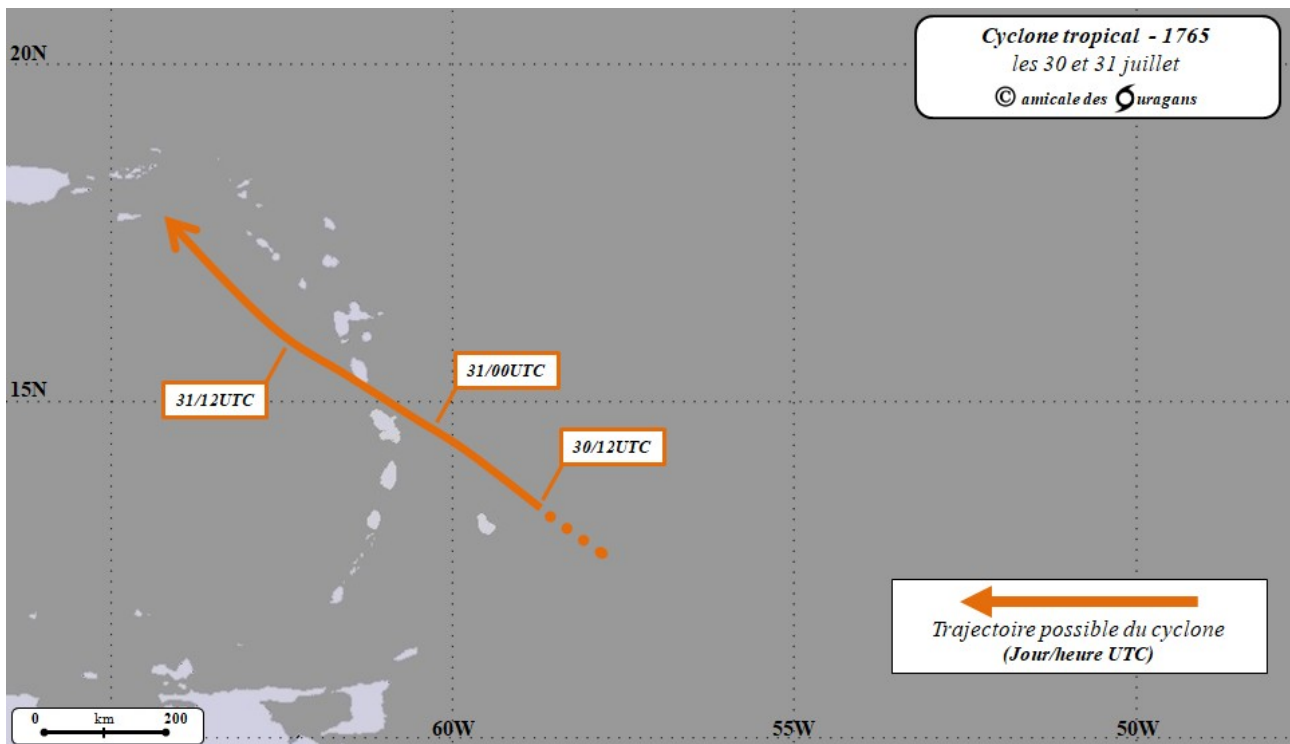
Trajectoire possible du centre du cyclone les 30 et 31 juillet 1765
